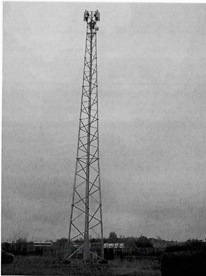
Załącznik nr 1: Widok ogólny instalacji radiokomunikacyjnej.
